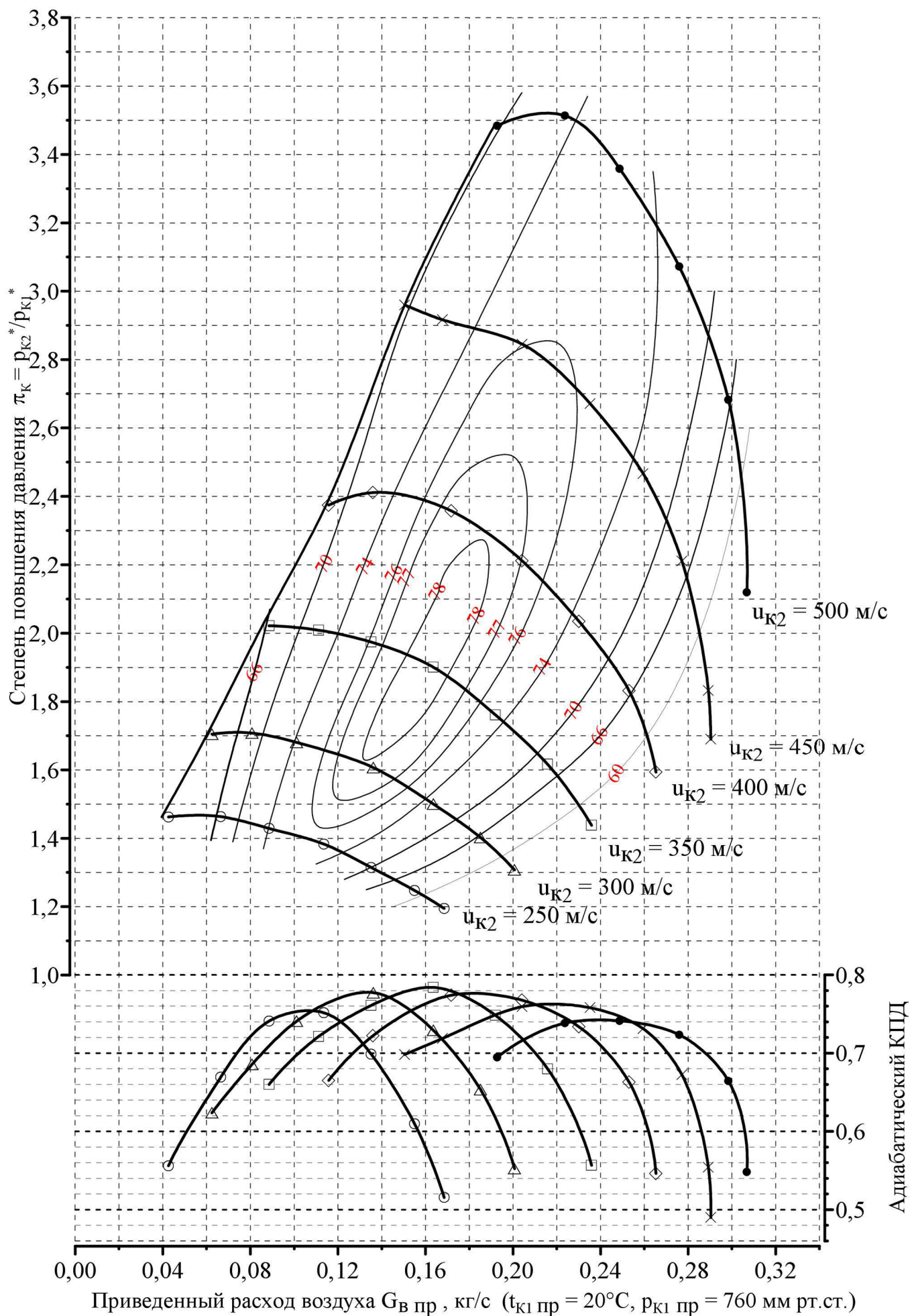
Характеристика компрессора ТКР 700.1-01, 700.1-02
